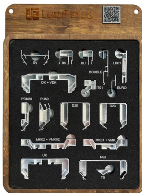
Профильный планшет LumFer silver
