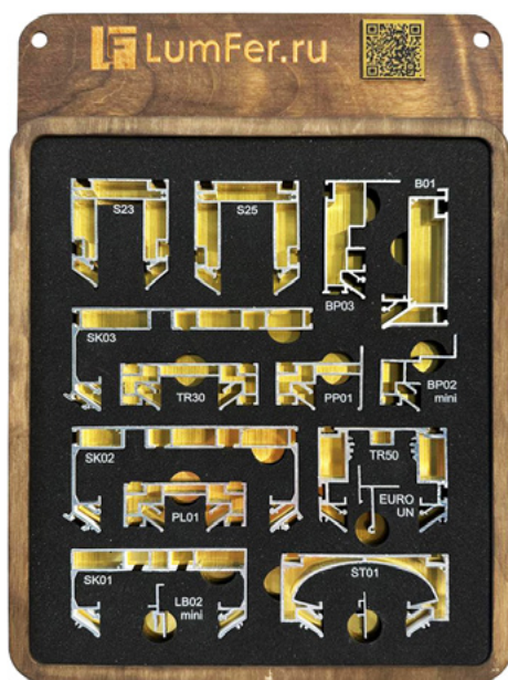
Профильный планшет LumFer gold
